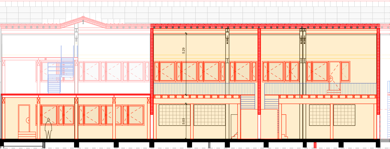
Schnitt AA
