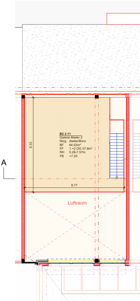
B2 2.11 Galerie: 64,02 m2
