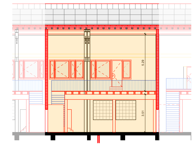
Schnitt AA
